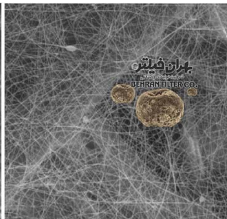
ساختار درونی کاغذ یک فیلتر هوای شرکت بهران فیلتر با فناوری نانوالیاف و عدم امکان عبور ذرات از میان حفرات آن
